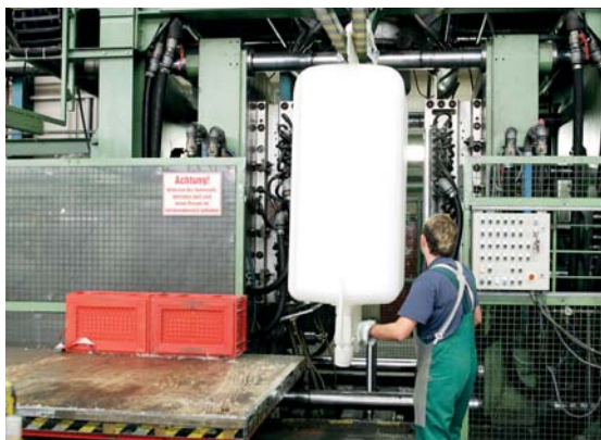
Blasformen
