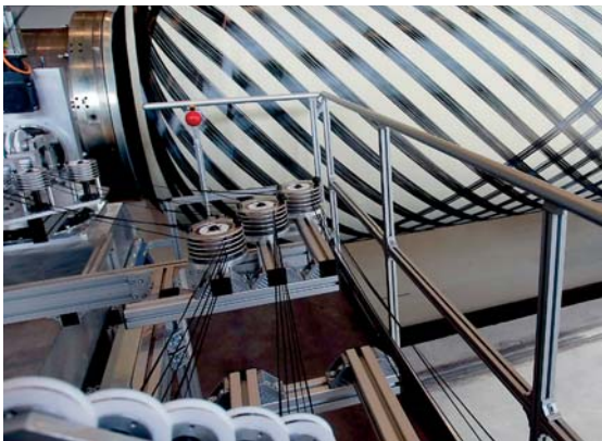
Detailansicht Wicklung
